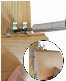
fissare il clip sulla sottostruttura
